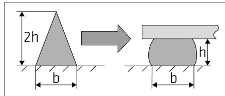
Figura 1: Compresión del cordón del adhesivo al tamaño final
